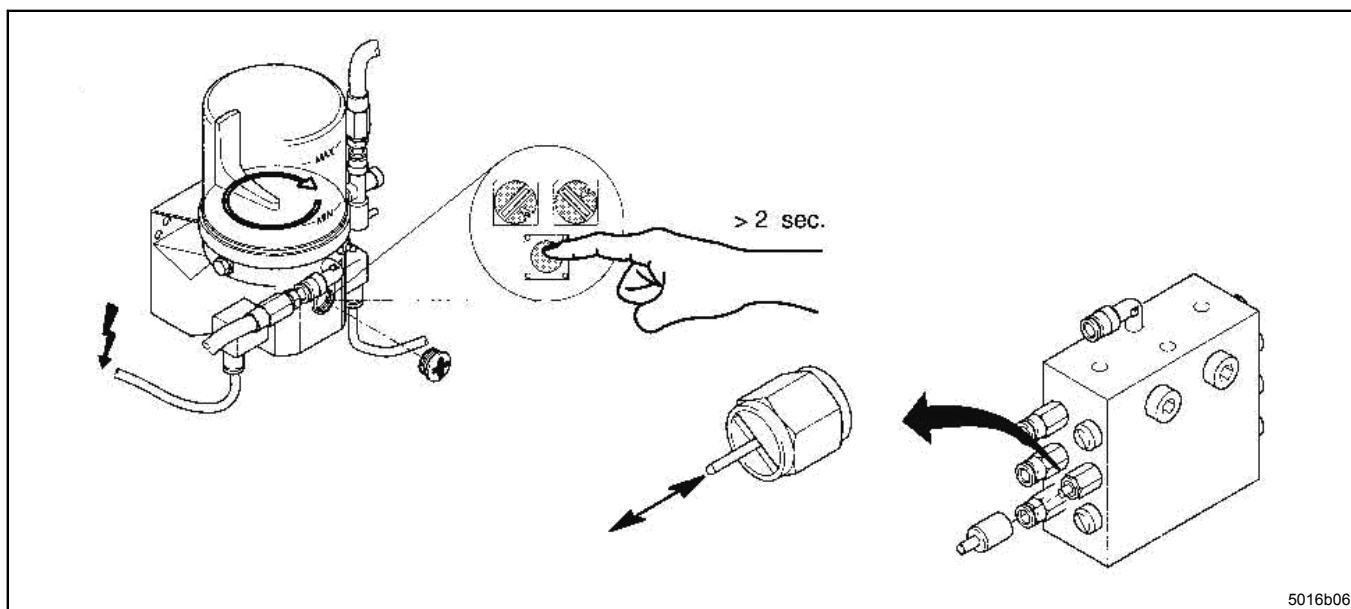
Рис. 19 Контроль работы насоса
