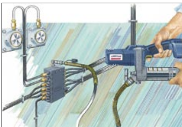
Централизованная система смазки Несколько смазочных точек объединяются в одну группу, подача смазочного материала, к которой осуществляется от одной точки
